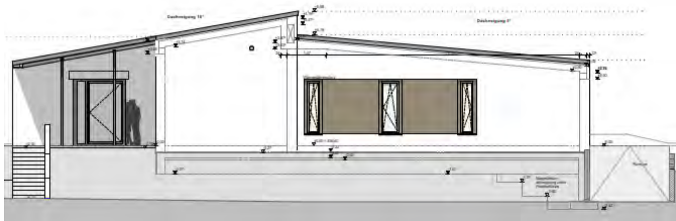
Ansicht Süd-West
